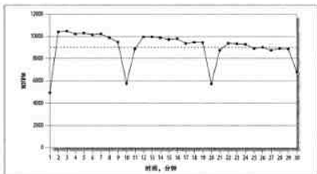
图2-3。一个30分钟的dbt2测试的结果
