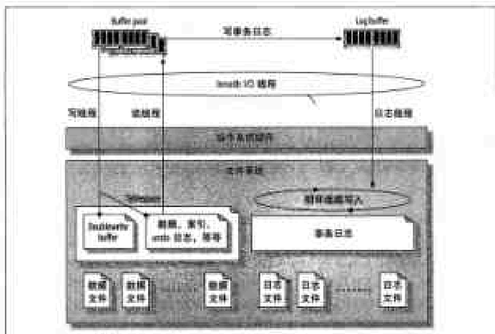
图5-1. InnoDB的缓存和文件
