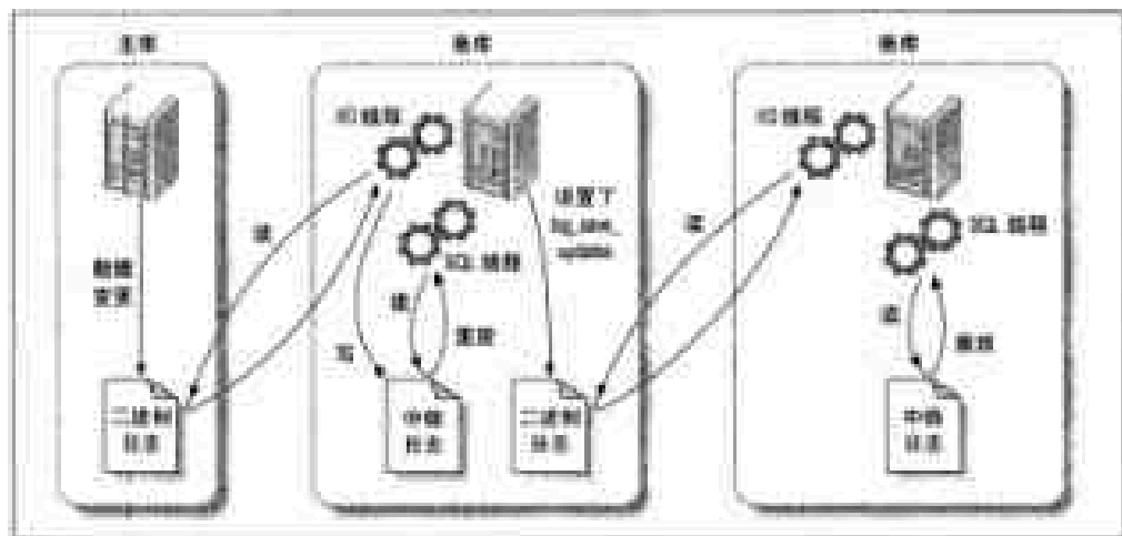
图10-2：将复制事件传递到更多的备库
