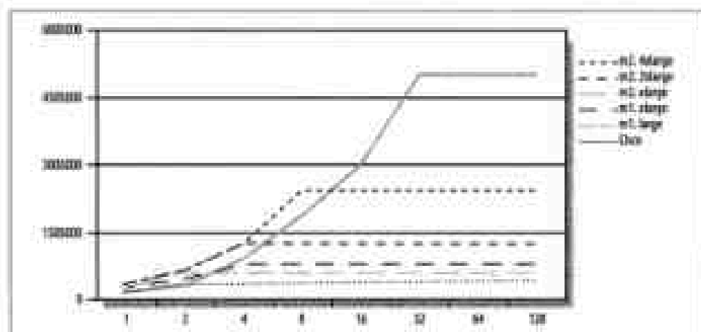
图13-2: 使用SysBench对AWS服务器进行CPU函数基准测试
