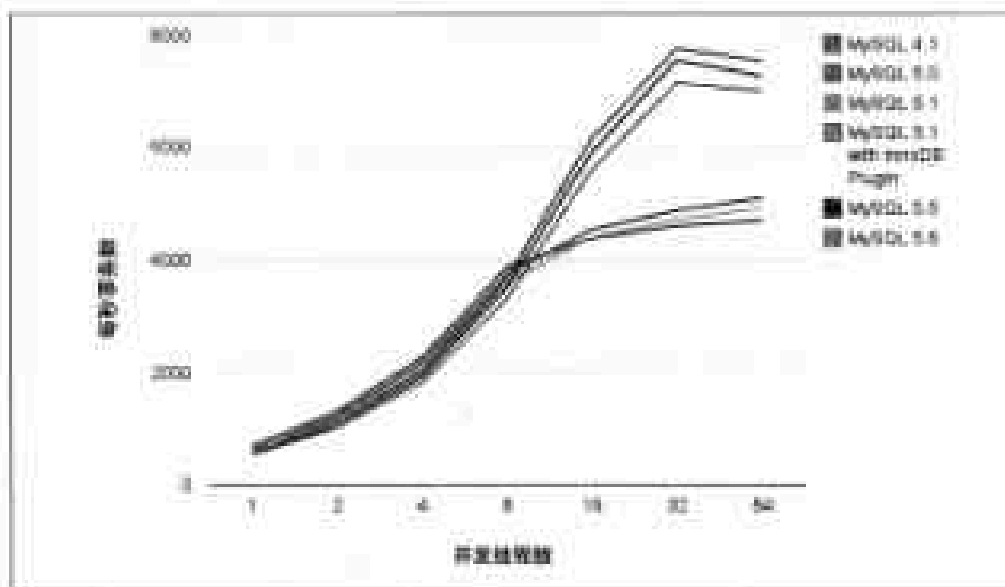
图 1-2, MySQL 不同版本的只读基准测试
