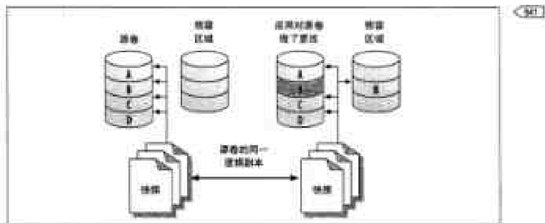
图 15-1，写时复制技术如何减少单个卷快照需要的大小
