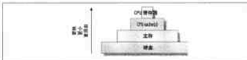
图 9-1 缓存层级
